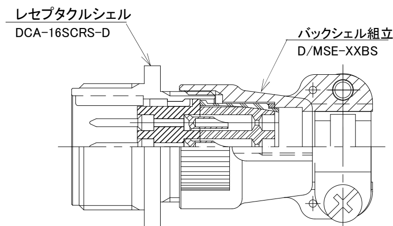
ケーブルレセプタクルコネクタ D/MS3101EXX-XXPXX
