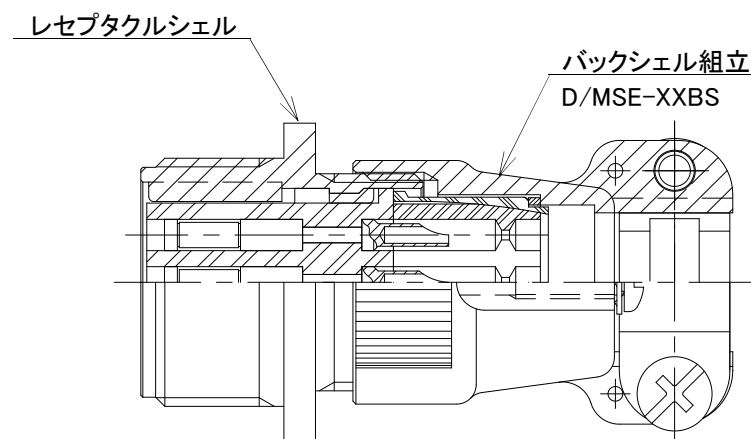
ケーブルレセプタクルコネクタ D/MS3100EXX-XXSXX
